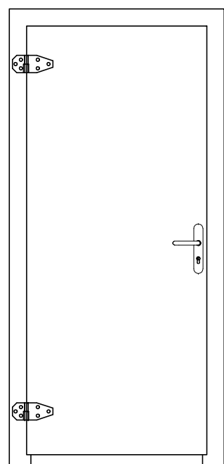
Drzwi rozwierane jednoskrzydłowe do hal produkcyjnych Wykonane ze stali nierdzewnej, wypełnione pianką PUR
