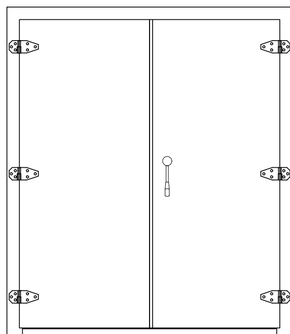
Drzwi rozwierane dwuskrzydłowe chłodnicze Wykonane ze stali nierdzewnej, wypełnione pianką PUR
