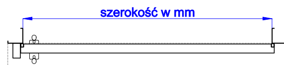
Drzwi rozwierane jednoskrzydłowe chłodnicze Wykonane ze stali nierdzewnej, wypełnione pianką PUR
