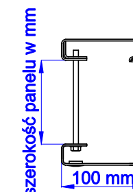
Ościeznica typu U (montaż do panelu)
